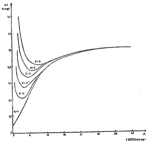
Figura 3: Atraso Médio Fim-A-Fim vs Taxa Média de Chegada para o Modelo Quarentena Local Semi-Duplex.
