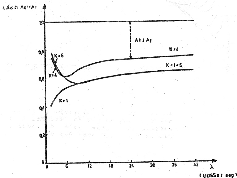
Figura 4: Participação das Medidas Atraso Médio de Admissão e Atraso Médio de Quarentena na Medida atraso Médio Fim-A-Fim para o Modelo Quarentena Local Semi-Duplex.
