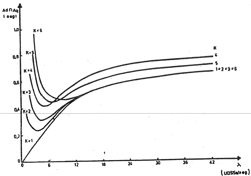
Figura 2: Atraso Médio de Admissão e Atraso Médio de Quarentena vs Taxa Média de Chegada de UDSSs para o Modelo Quarentena Local Semi-Duplex.
